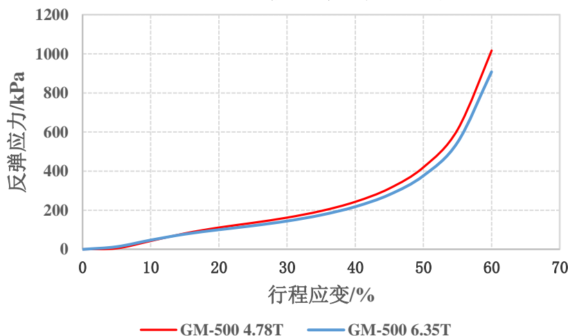
GM-500压缩反弹应力曲线
