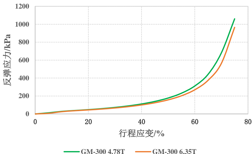
GM-300压缩反弹应力曲线
